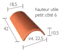
Faîtère/arêtier de 42 à recouvrement (± 2,8/ml)
