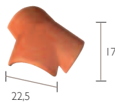
Rencontre 3 voies Pente < 50 %
