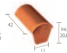
Faîtère d'about de 42 (fin) (Fixation obligatoire)
