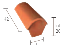
Faîtère d'about de 42 (début) (Fixation obligatoire)
