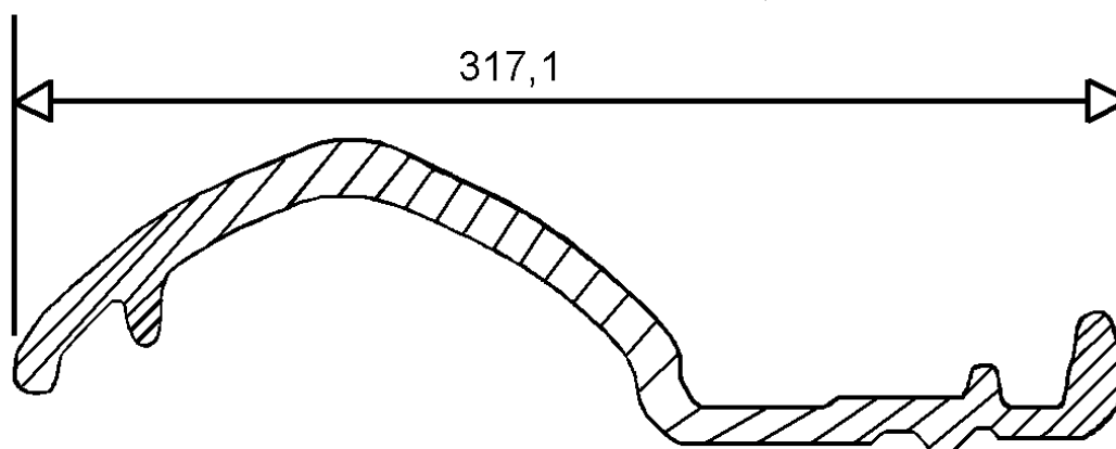
Figure 1 – Coupe longitudinale
