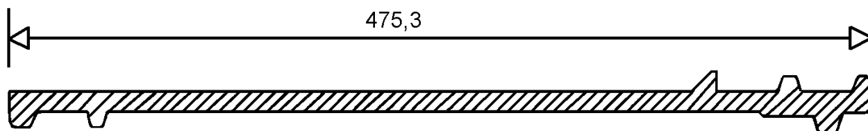
Figure 1 – Coupe longitudinale
