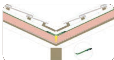
TRAITEMENT DE LA NOUE
