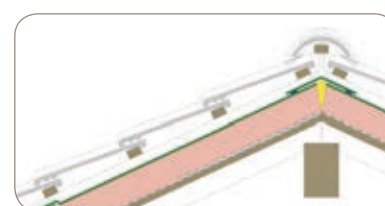
TRAITEMENT DU FAÎTAGE
