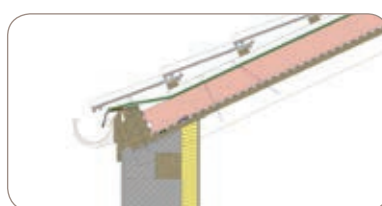
TRAITEMENT DE L'ÉGOUT
